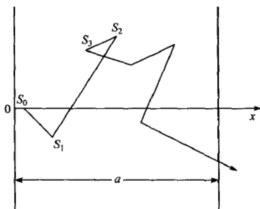
图 3.7.1 中子穿越物质层模拟示意图
