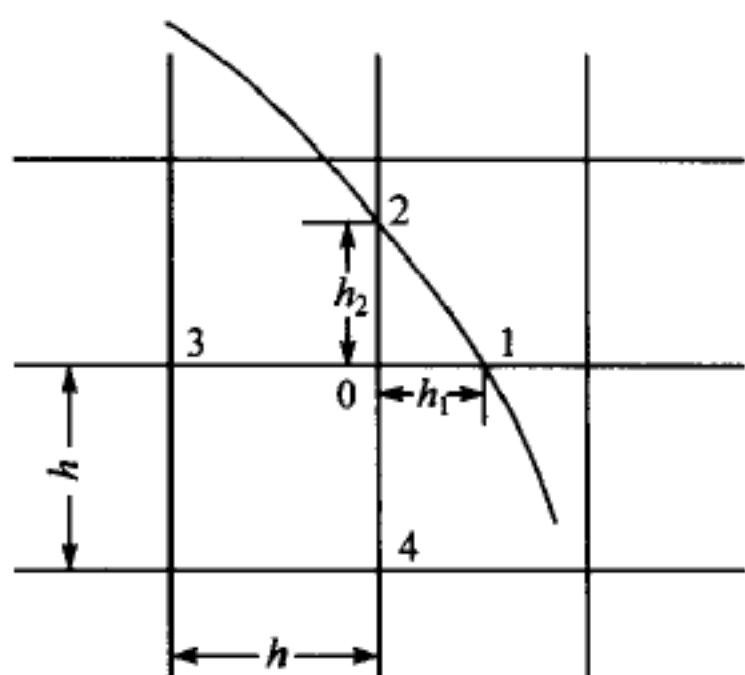
图 4.2.4 场域的第一类边界条件
