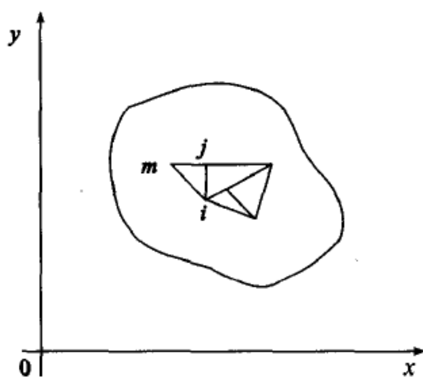
图 5.2.2 不允许的三角形元素的划分
