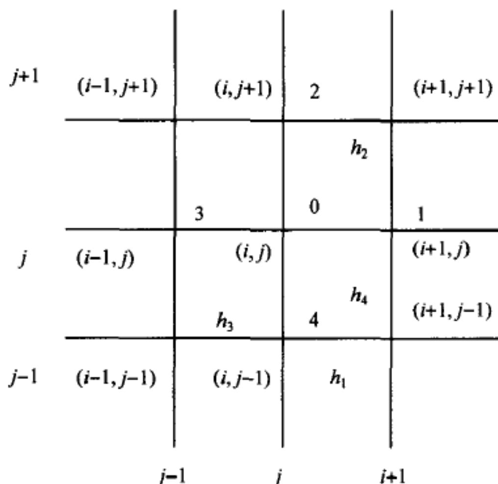
图 4.1.1 节点 0 及邻近节点
