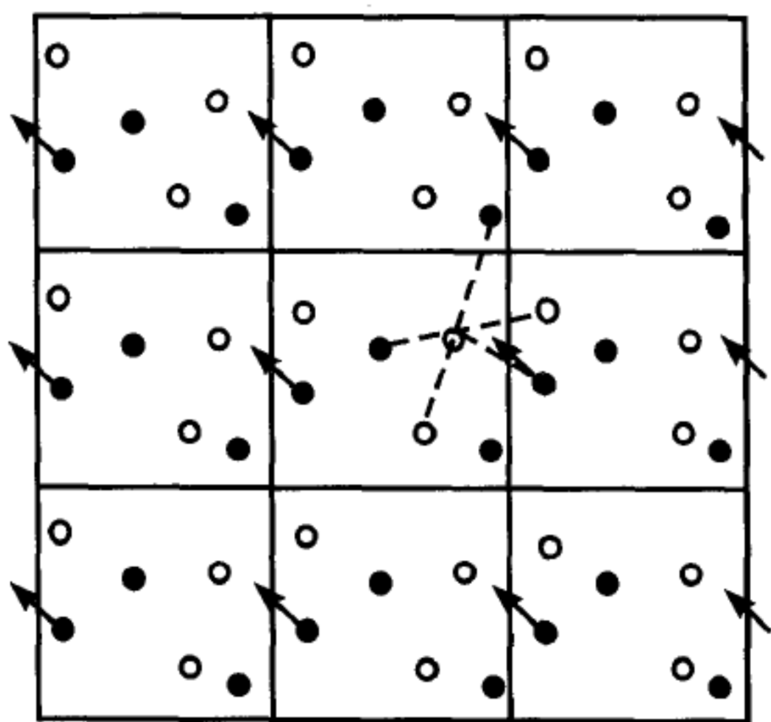
图 6.2.1 分子动力学模拟的最小像力约定
