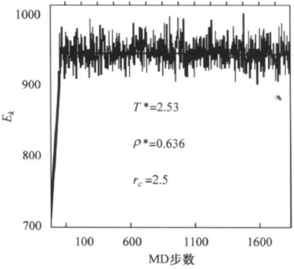
图 6.4.1 动能演化过程图( T^* = 2.53 )
