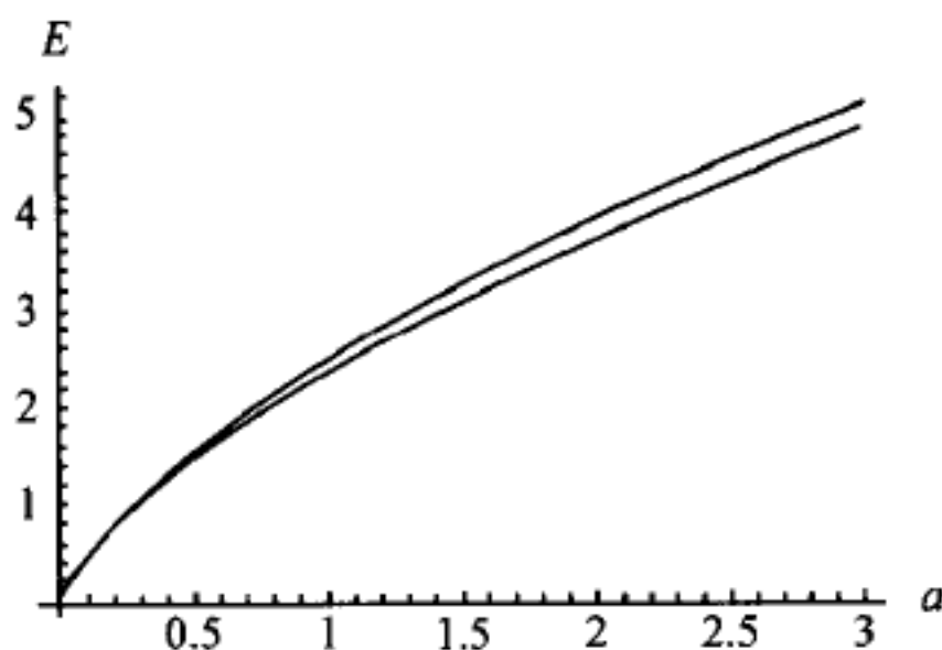
图 8.2.4 线性势基态能量真值和变分上限
