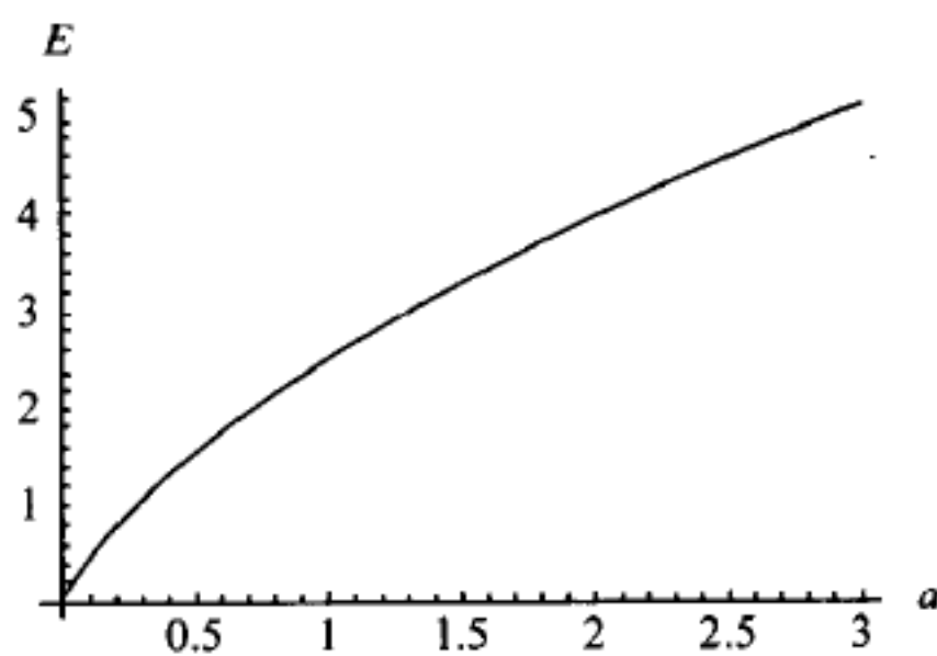
图 8.2.3 线性势基态的变分上限 能量 E_{\text{var}}
