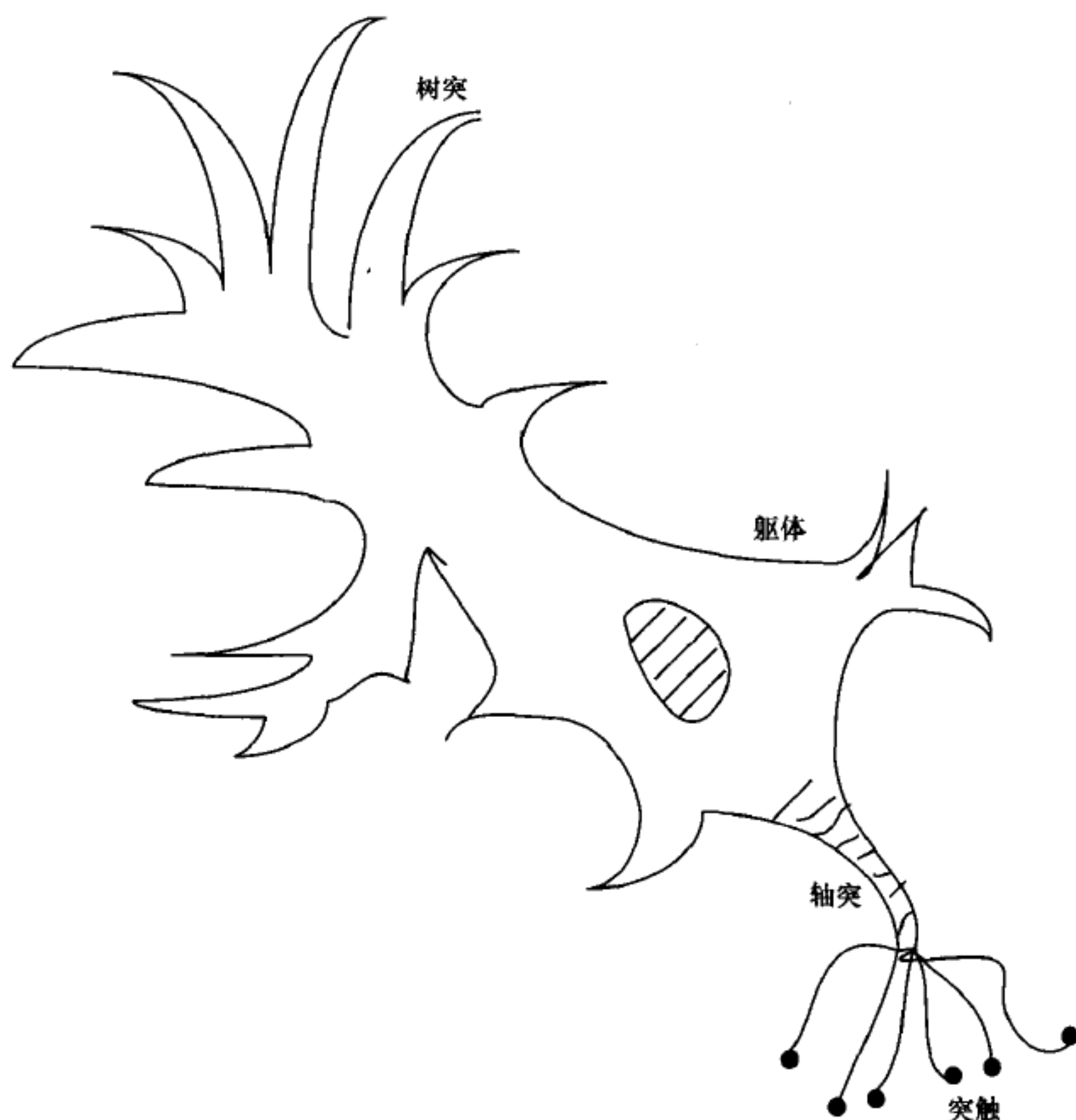
图 9.1.1 神经元基本结构
