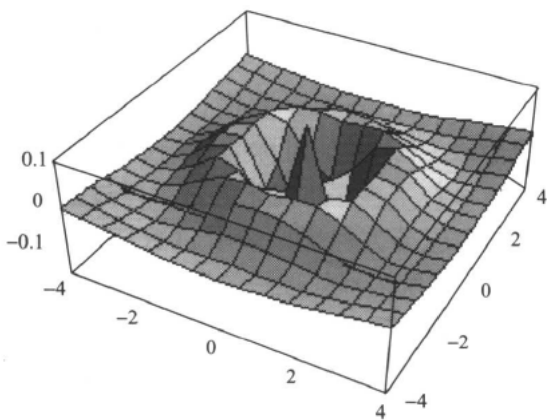
图 8.2.6 k=5 且 l=m=0 时的“试探”波函数 \phi_{k,lm}(x, y)
