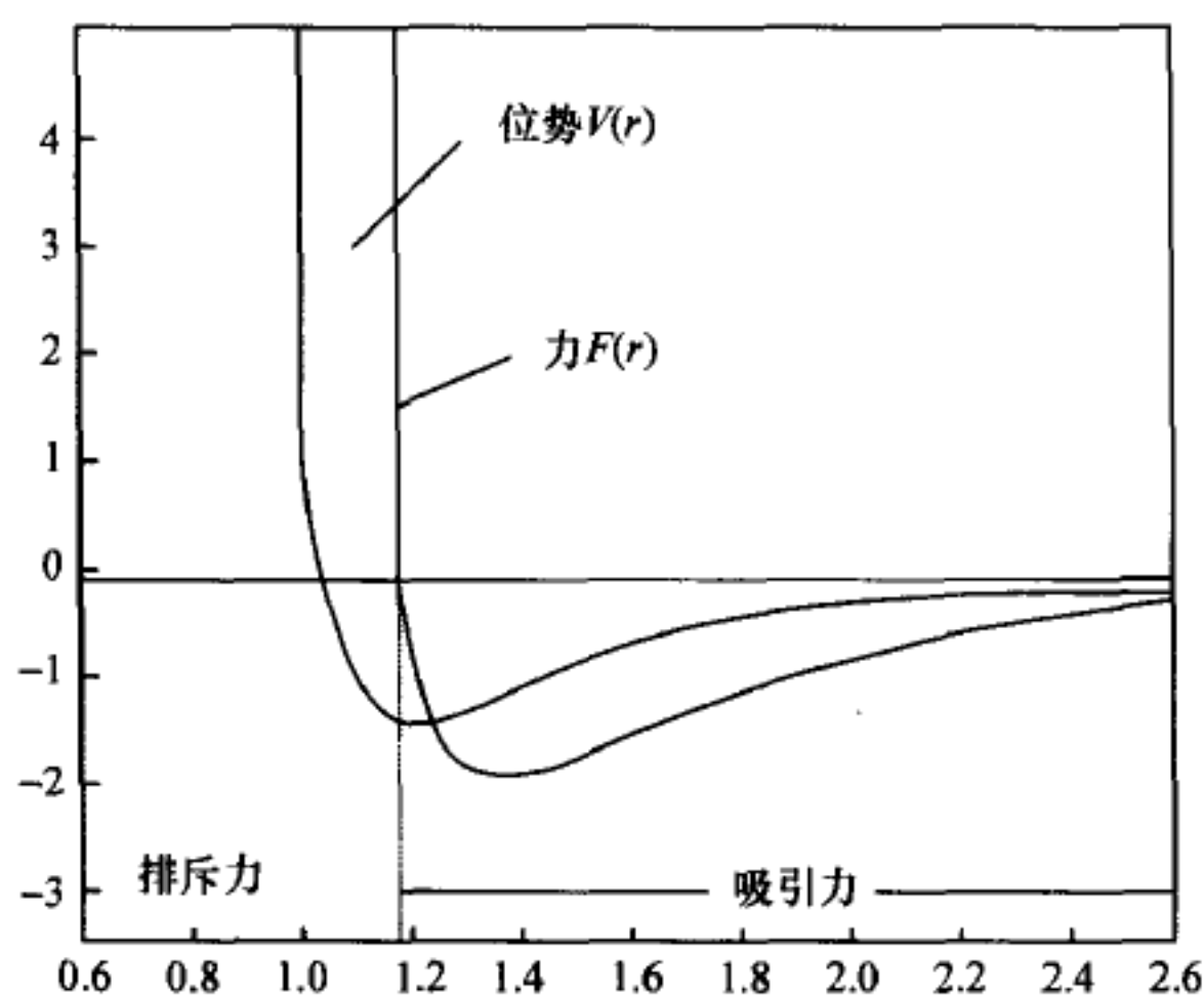
图 6.3.1 Lennard-Jones 势
