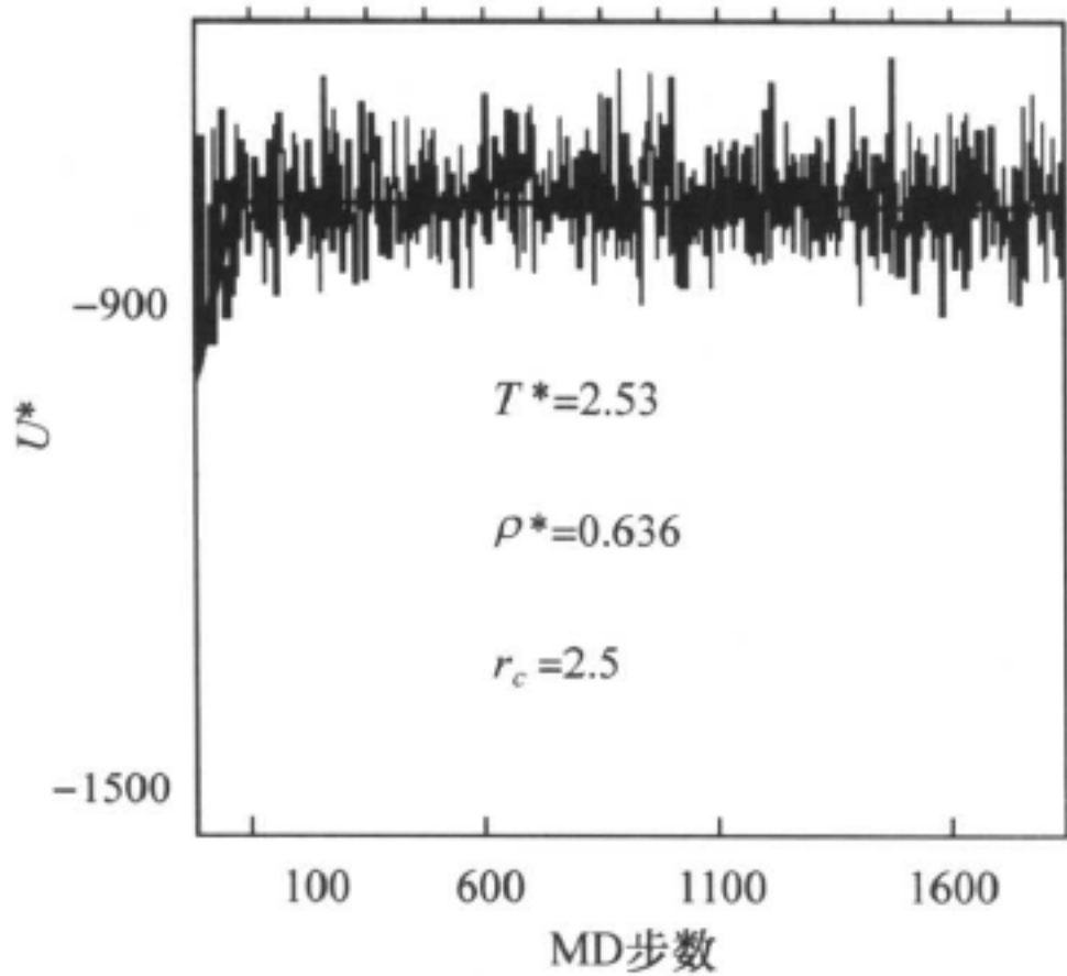
图 6.4.2 位能演化过程图( T^* = 2.53 )
