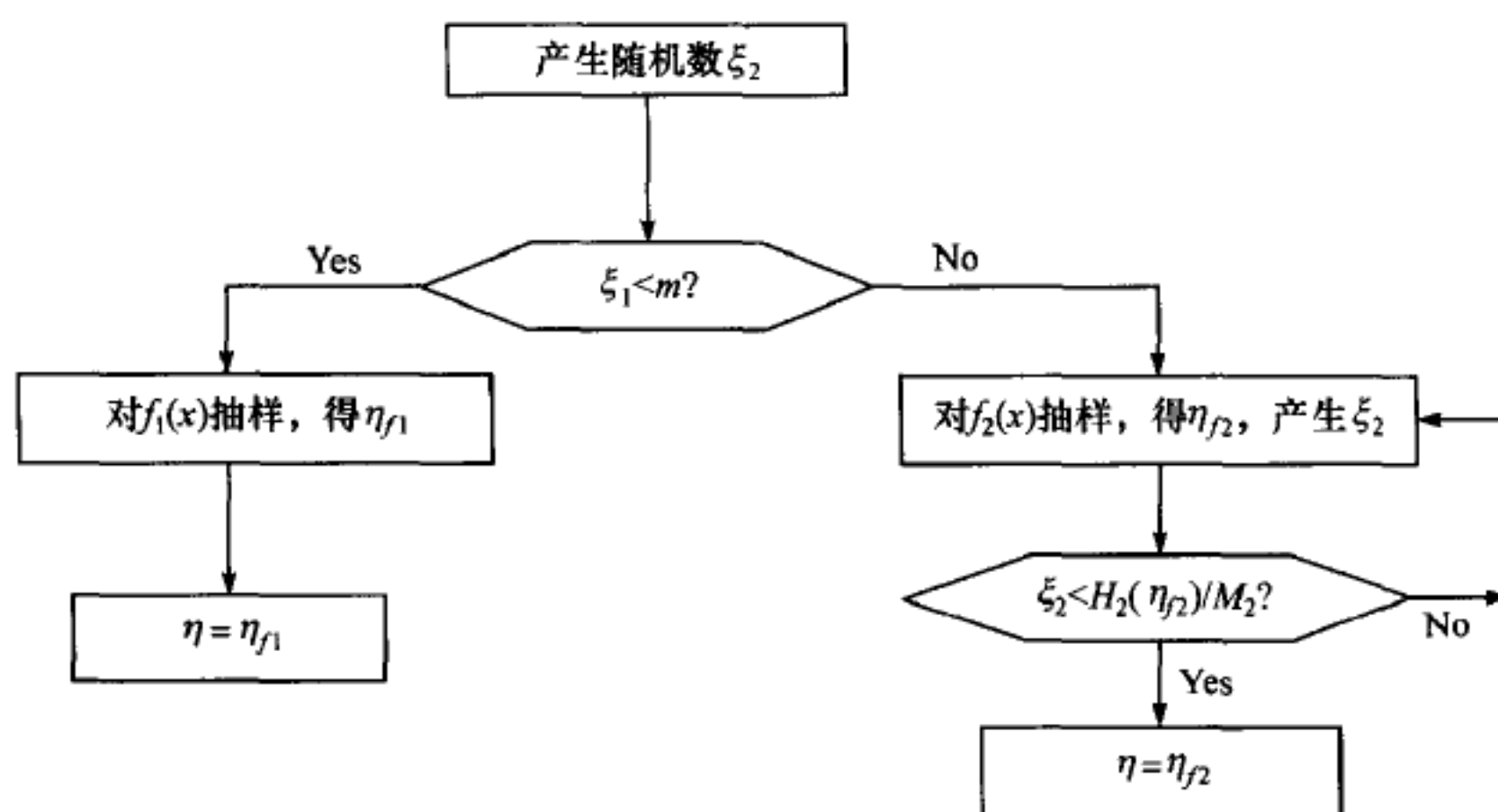
图 2.3.3 近似修正抽样框图
