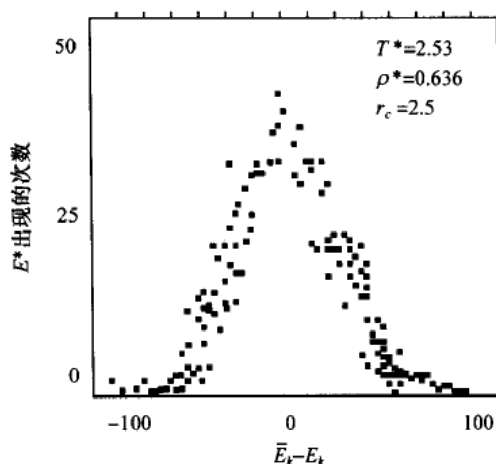
图 6.4.4 动能的分布图( T^* = 2.53 )
