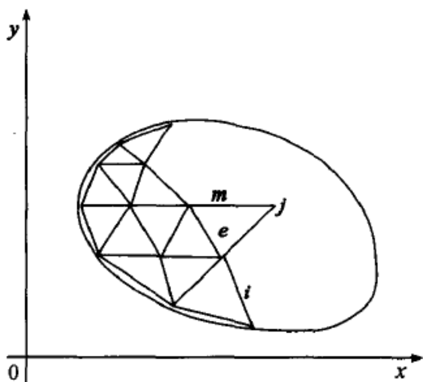
图 5.2.1 允许的三角形元素的划分
