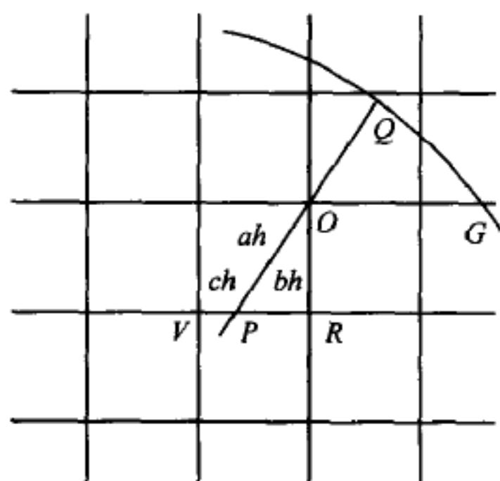
图 4.2.5 场域的混合边界条件
