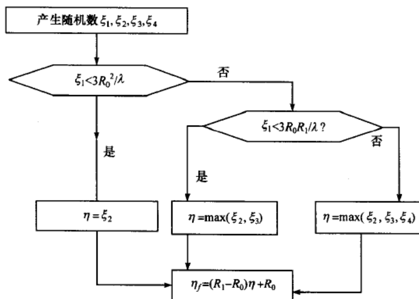
图 2.3.2 球壳均匀分布的抽样图
