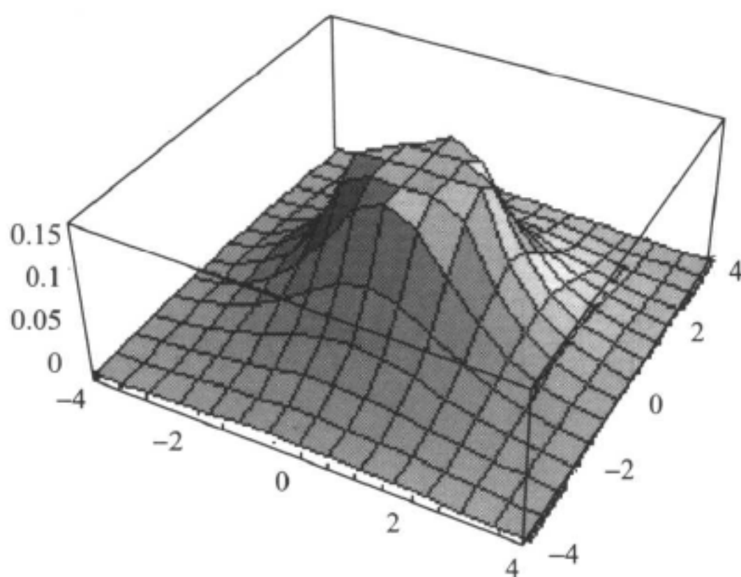
图 8.2.5 k=l=m=0 时的“试探”波函数 \phi_{k,lm}(x, y)
