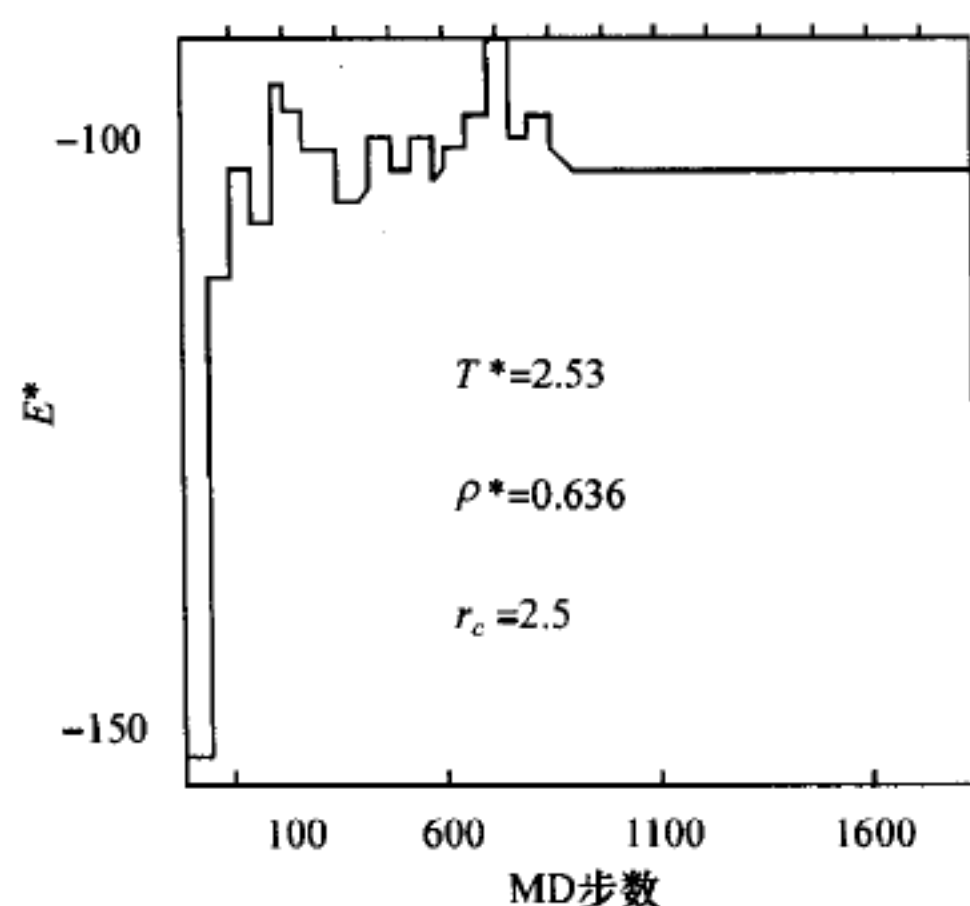
图 6.4.3 总能量演化过程图( T^* = 2.53 )
